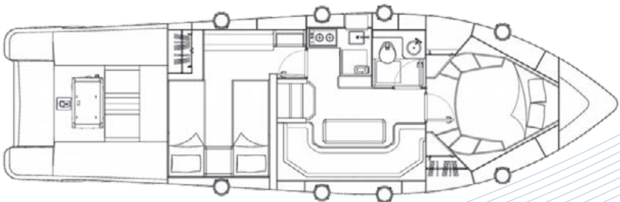
CONVÉS INFERIOR
