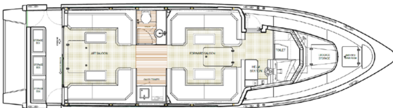
PLAN DU PONT(LOUNGE)
