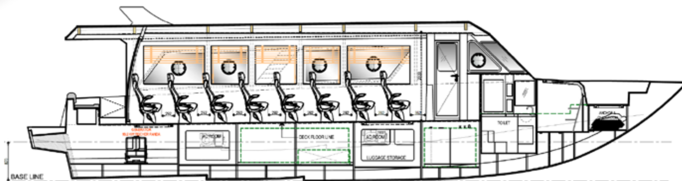
SECCIÓN INTERIOR (STBD)
