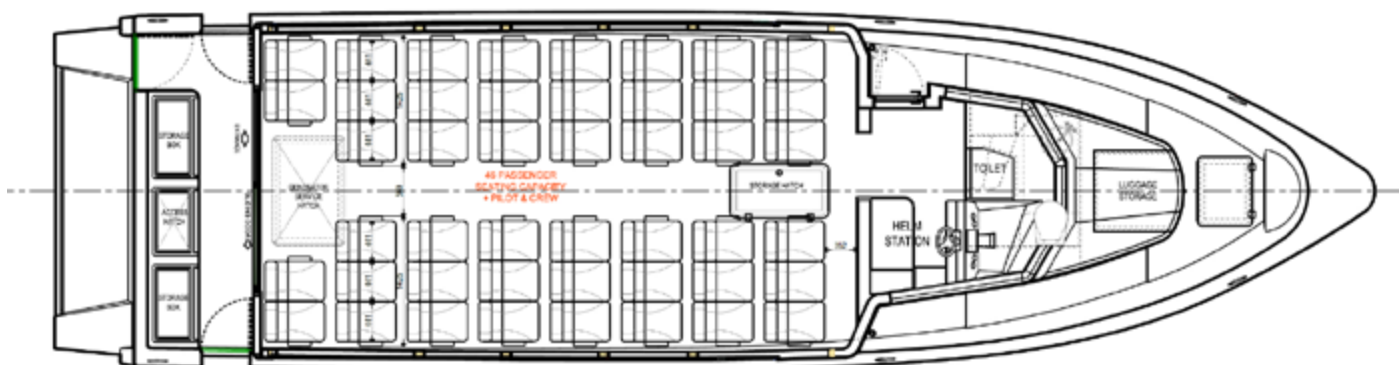
PLANO DE LA CUBIERTA (VERSIÓN DE PASAJEROS)
