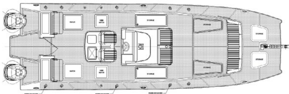
PLAN DU PONT
