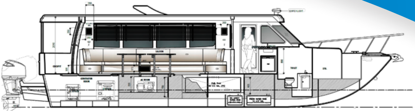
SECCIÓN DE LA ENTRECUBIERTA
