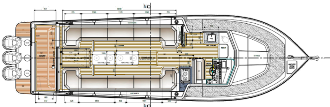
DISTRIBUCIÓN GENERAL
