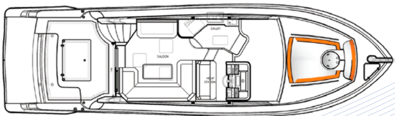
PLANO DE CUBIERTA
